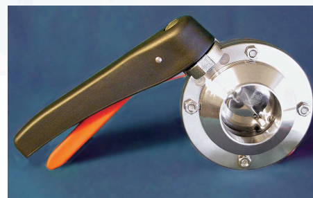
Spjällventil
